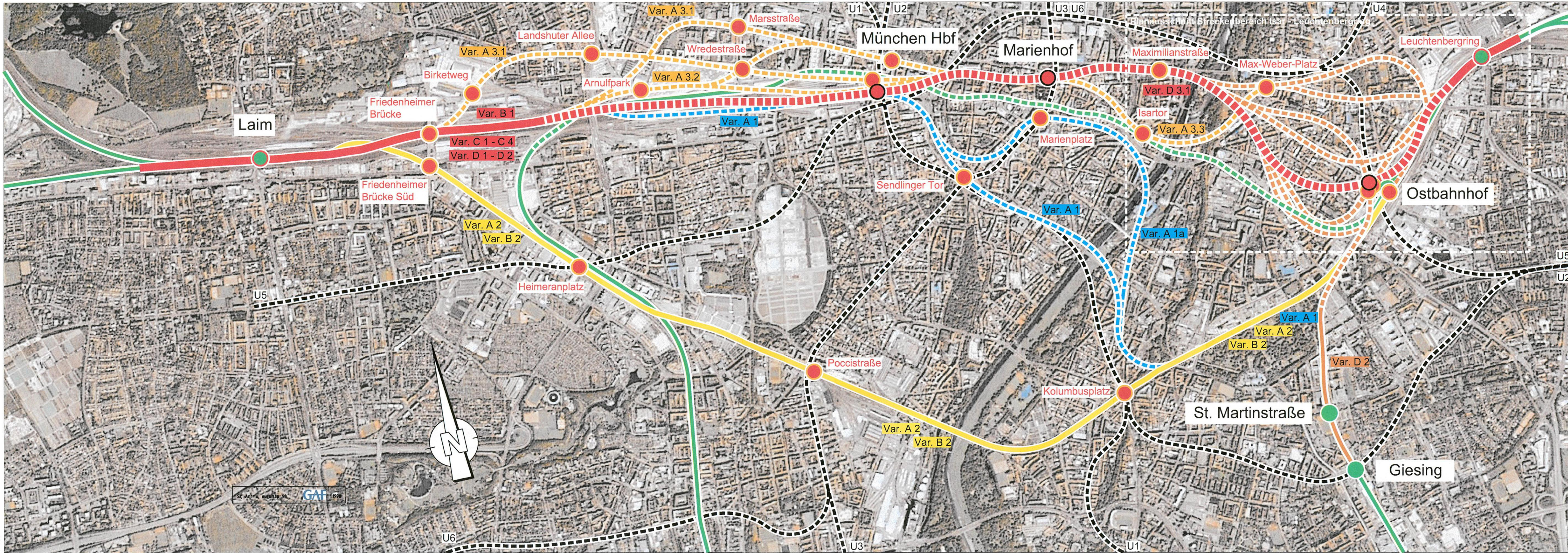
Planausschnitt Streckenbereich Isar - Leuchtenberg
