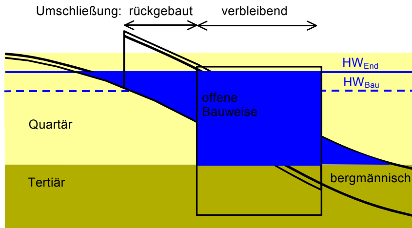
Abb. 10.1: Schemadarstellung Tunnelbauwerk im quartären Grundwasser bei HW_{End}
